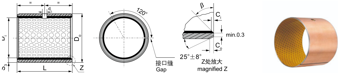
内外倒角 ID and OD chamfers
